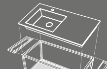
Era 100 Struttura sospesa Wall-hung framework cm 100 x 46 x 40 h
