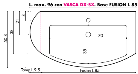
Art. F309 Per basi portalavabo Fusion L 85 cm P. 280
