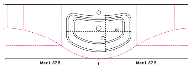
Art. F701 Per basi portalavabo min. L 70 x P 50 cm P. 281
