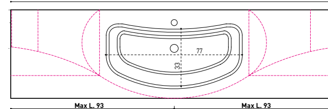
Art. F702 Per basi portalavabo min. L 85 x P 50 cm P. 281
