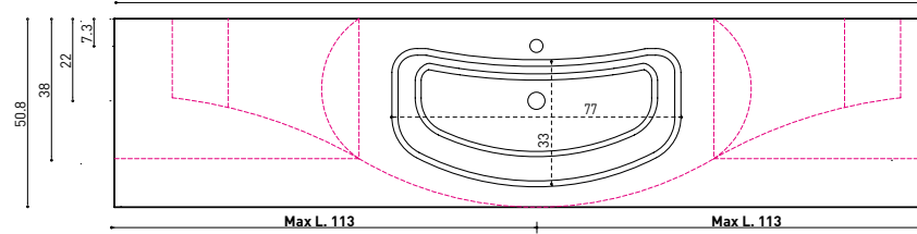
Art. F802 Per basi portalavabo min. L 85 x P 50 cm P. 281
