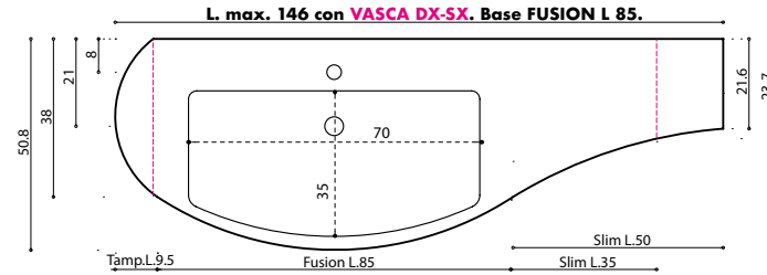
Art. F308 Per basi portalavabo Fusion L 85 cm P. 280
