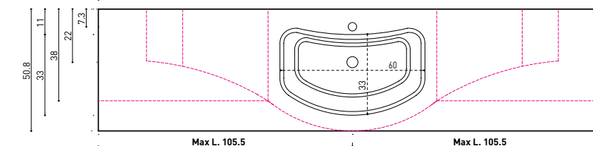
Art. F801 Per basi portalavabo min. L 70 x P 50 cm P. 281
