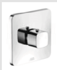
термостат, скрытый монтаж # 11730000 термостат Highflow, скрытый монтаж # 11731000 скрытая часть iBox® universal (без рис.) # 01800000
